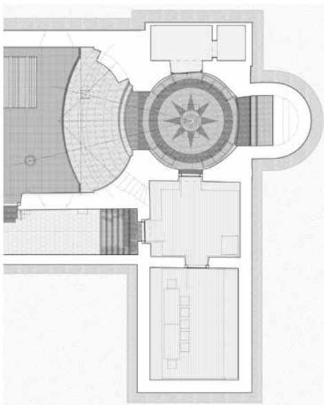
5. kép Az új, megemelt ambó terének kialakítása és alaprajzi szerkesztése a centrális tér kiterjesztéseként. (Hetedik Múterem Kft.)
